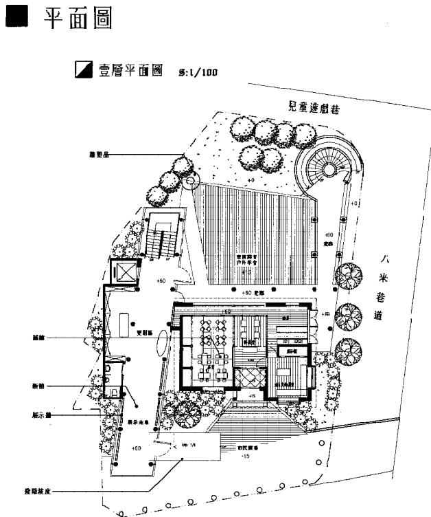
圖1&2 文山公民會館規劃設計案配置圖與平面圖(孫啟榕建築師事務所)
